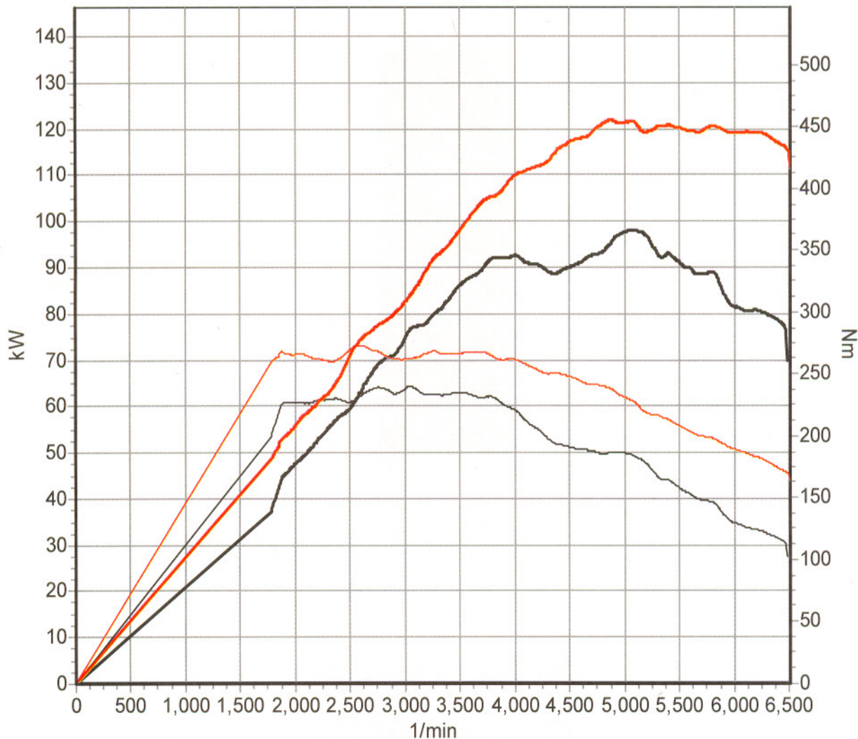
P-max Motorleistung (gem.) / Geschwindigkeit / Drehmoment (gem.)
